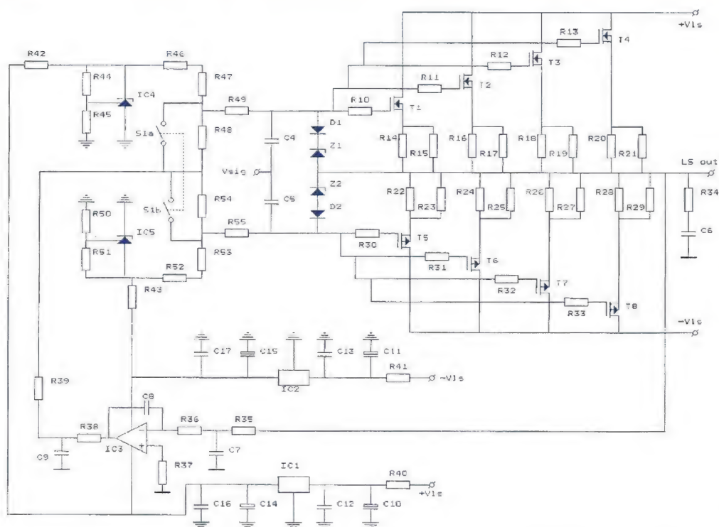
Figuur 2 De stroomversterker
